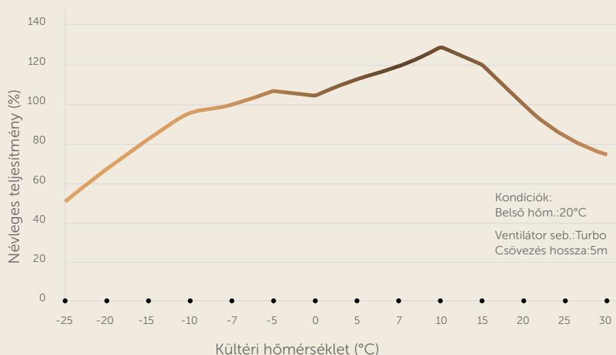
2,5 és 3,5 kW-os Comfort Pro fűtési teljesítménye különböző külső hőmérsékletek mellett
